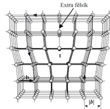
Éldiszlokáció (1D) Csavardiszlokáció (1D) Vegyes (1D)
