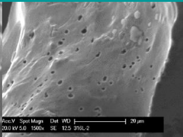
316L lyukkorrózió
