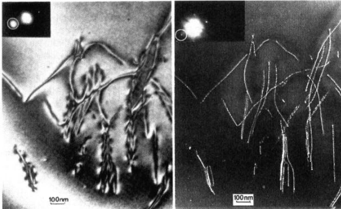
Diszlokációk Si-ban
