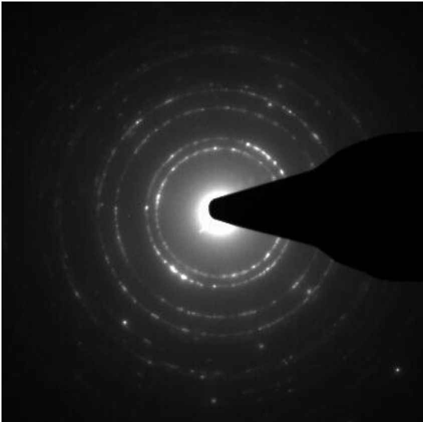
Diffrakciós kép
