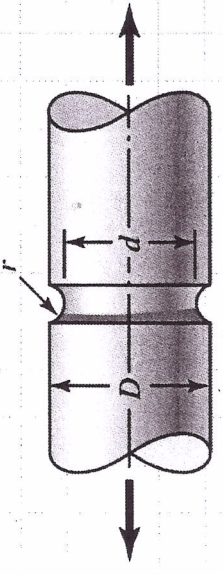
FESZÜLTÉGKONCENTRÁCIÓS TÉNYEZŐ ÉRTÉKEI HÚZOTT BEMETSZETT HENGERRE ( r/D 0,050 - 1,000)
