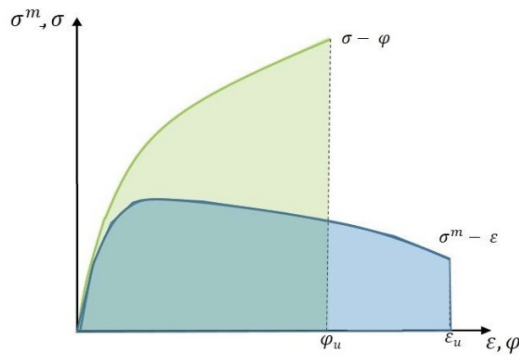
A fajlagos törésmunka grafikus értelmezése mérnöki és valódi rendszerben.
