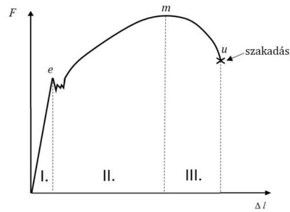
Egy lágycélra jellemző szakítódiaagram a jellemző szakaszok bejelölésével
