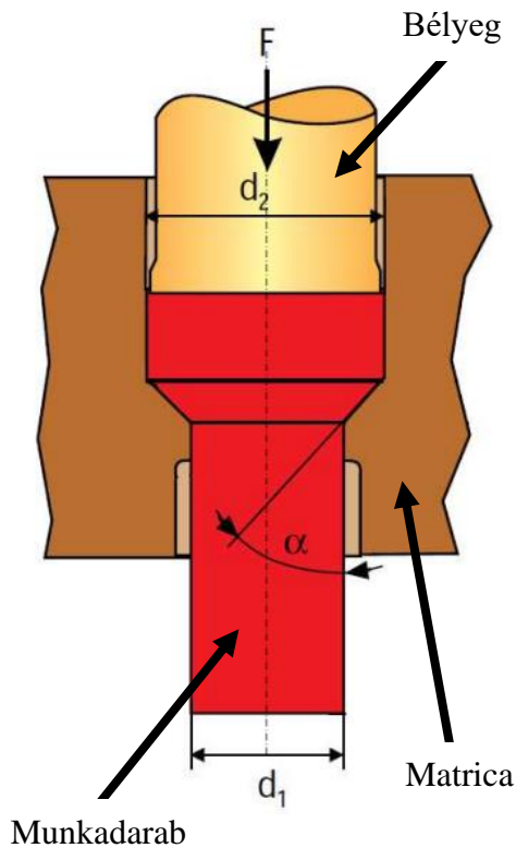
5. ábra. Az előrefolytatás sematikus ábrája
