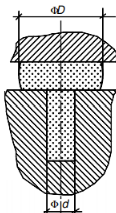
7. ábra. Csavar fejrészének elkészítése folyatással, majd fejezéssel.
