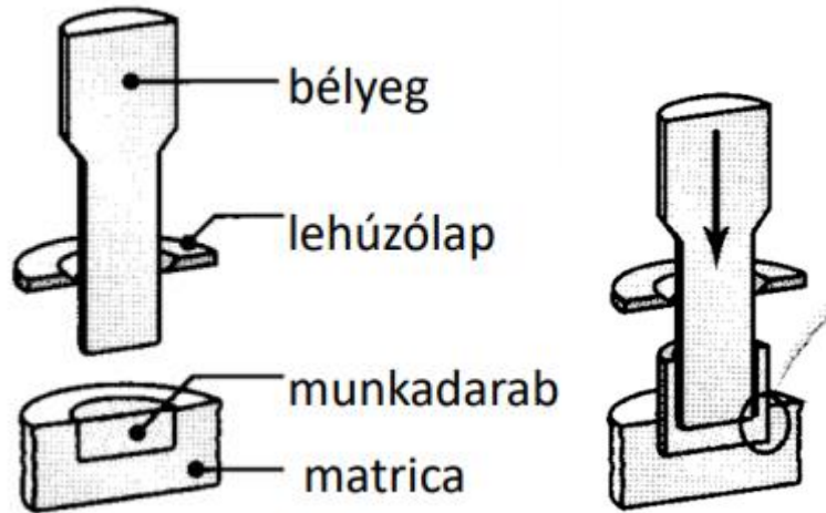
6. ábra. A hátrafolytatás sematikus ábrája
